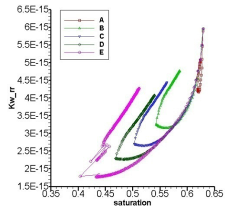
شکل ۱۱: تغییرات نفوذپذیری (با واحد متر بر ثانیه) نسبت به درجه اشباع برای المانی نزدیک به منبع حرارتی در نمونه پینتادو روند کاهشی نفوذپذیری می‌شود. زمانی که منبع حرارتی قطع می‌شود، مقدار شکست ثابت می‌ماند ولی جهت جریان آب در نمونه عوض می‌شود و درجه اشباع در این المان افزایش می‌یابد، در نتیجه نفوذپذیری افزایش می‌یابد.
