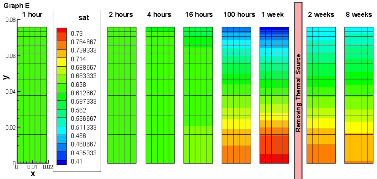
شکل ۴: خطوط هم تراز درجه اشباع برای گراف E در نمونه پینتادو
