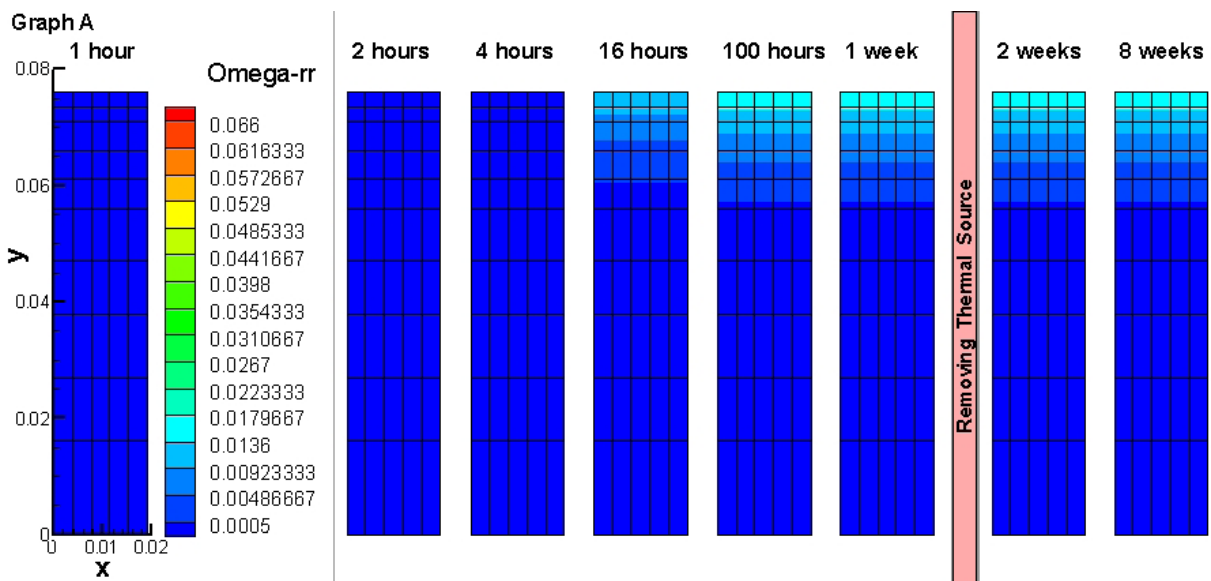
شکل ۵: خطوط هم تراز عامل شکست برای گراف A در نمونه پینتادو
