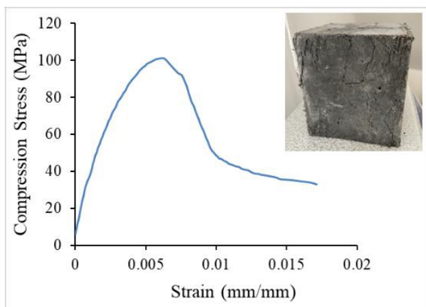
شکل ۶. منحنی ایده‌آل تنش-کرنش فشاری.
