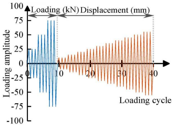
شکل ۱۱. نمودار بارگذاری چرخه‌ای جانبی [۵۸].
