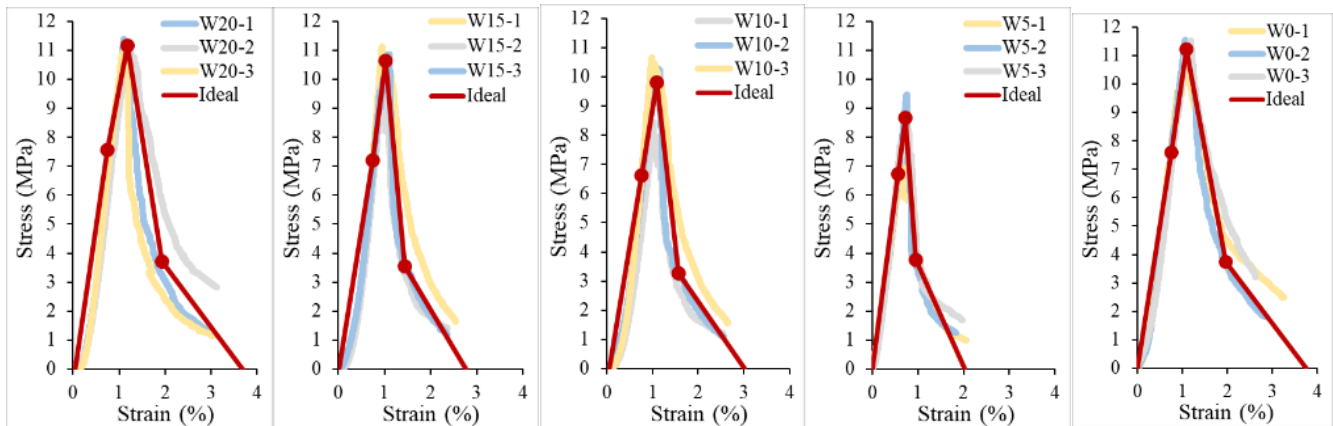
شکل ۴. نمودار تنش-کرنش آزمون‌های دمبلی شکل تحت کشش مستقیم به همراه منحنی ایده‌آل برای پنج ترکیب.
