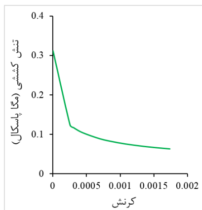
شکل ۹. نمودار تنش-کرنش کششی بتن.
