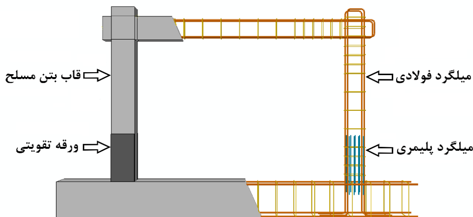
شکل ۱۵. جزئیات مدل عددی قاب‌های تقویت شده.
