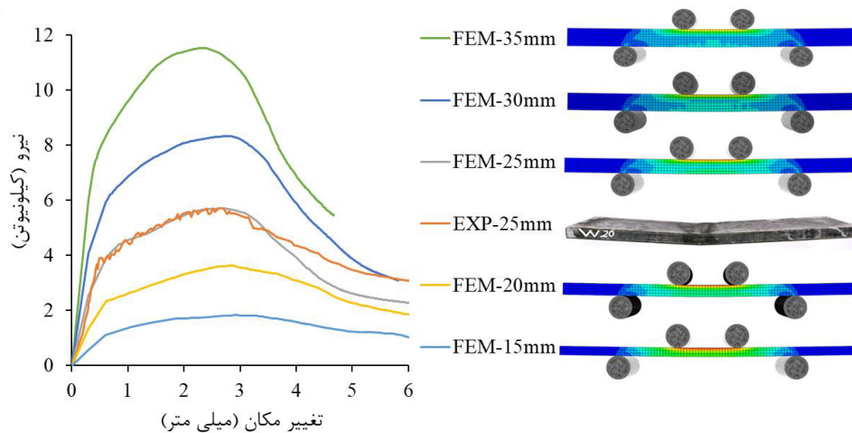
شکل ۱۴. نمودار نیرو-تغییر مکان آزمایش خمشی ورقه ۵۰۰ میلی متری به همراه مدل سازی عددی.
