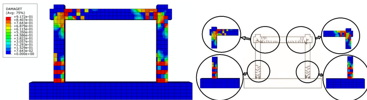
شکل ۱۳. خسارت کششی بتن در دهمین چرخه و مقایسه با قاب آزمایشگاهی.
