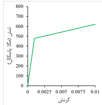
شکل ۱۰. نمودار تنش-کرنش میلگرد فولادی.
