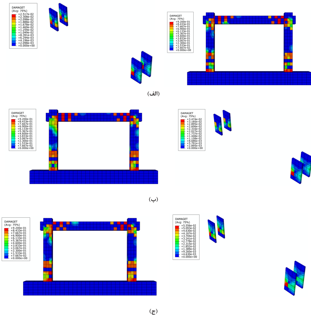
شکل ۱۸. خسارت کششی به همراه خسارت کششی ورقه در دهمین چرخه برای قاب‌های (الف) T35N4G12، (ب) T35N4G10، و (ج) T25N4G12.
