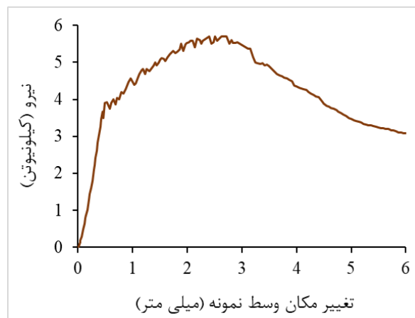
شکل ۵. نمودار نیرو-تغییر مکان آزمایش خمشی.
