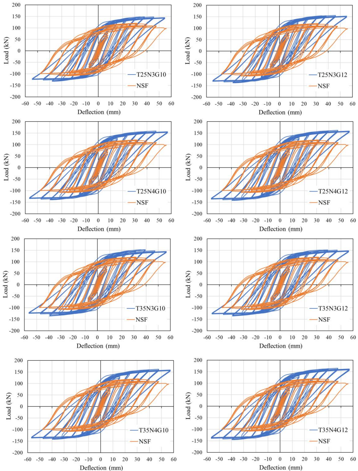
شکل ۱۶. نمودارهای نیرو-تغییر مکان برای قاب‌ها.
