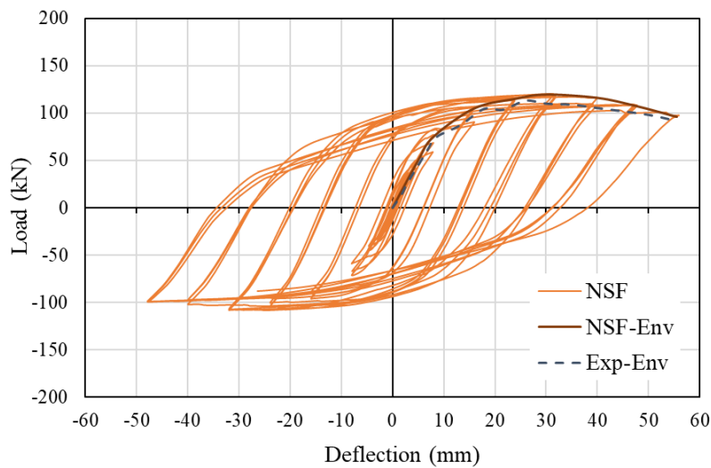
شکل ۱۲. نمودار بارگذاری چرخه‌ای جانبی [۵۸].
