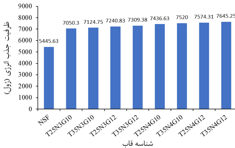
شکل ۲۰. ظرفیت جذب انرژی بر حسب نام اختصاری قاب‌ها.
