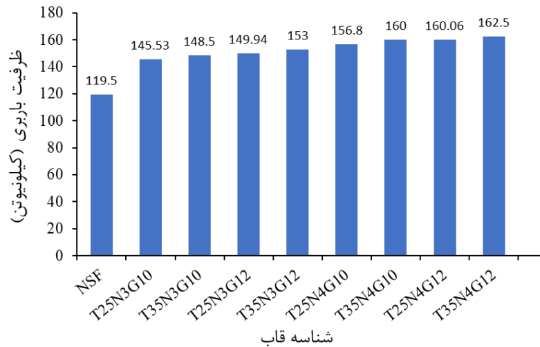
شکل ۱۹. ظرفیت باربری بر حسب نام اختصاری قاب‌ها.
