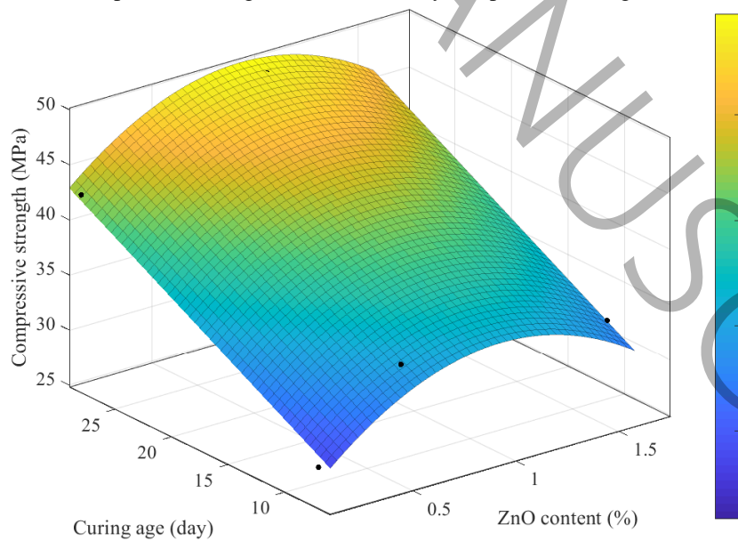
شکل ۱۳ آنالیز حساسیت سه بعدی مقاومت فشاری بتن بر اساس میزان نانوذرات و سن بتن Figure 13 Three-dimensional sensitivity analysis of concrete compressive strength based on the amount of nanoparticles and age of concrete
