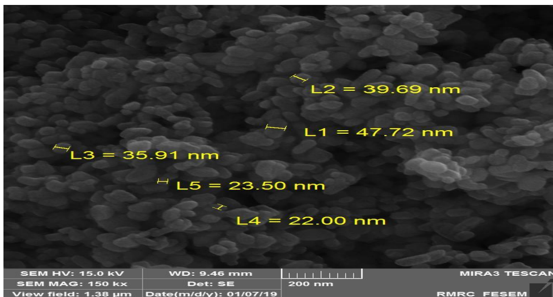
شکل ۳. SEM نانو ذرات دی اکسید تیتانیوم (TiO 2 )
