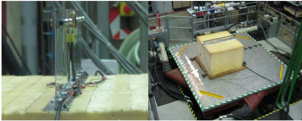
شکل ۲. نمونه‌ی آزمایشگاهی مطالعه شده توسط آلدایخ و همکاران [۱۸]
