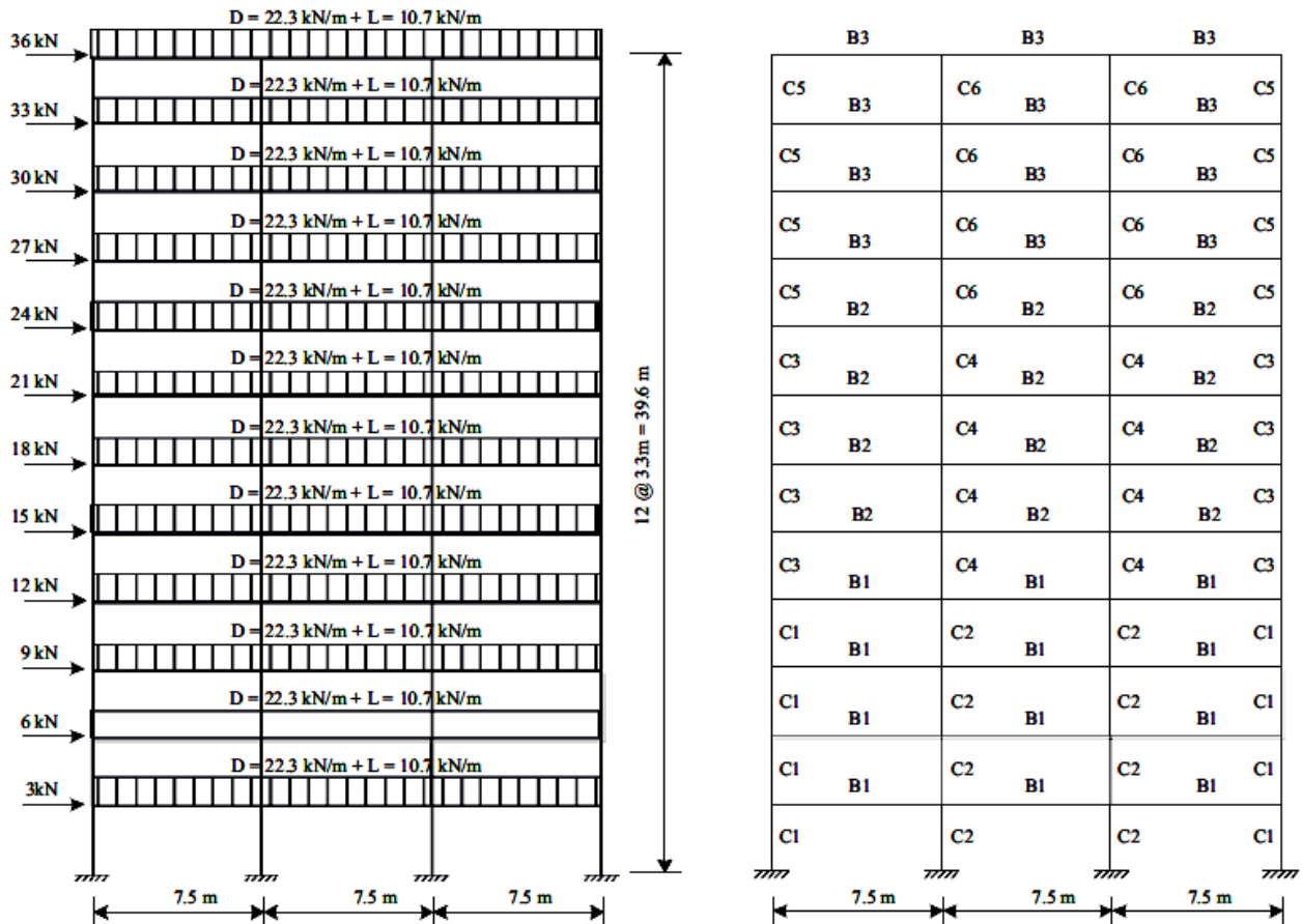
شکل ۸. هندسه، بارگذاری و گروه‌بندی اعضای ساختمان ۱۲ طبقه [۲۱]
