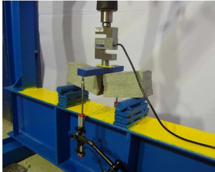
شکل ۵. نحوه انجام آزمایش خمش سه نقطه‌ای.
