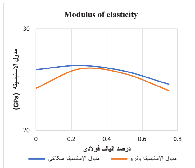
شکل ۲۷. منحنی مدول الاستیسیته طرح های دارای الیاف فولادی
