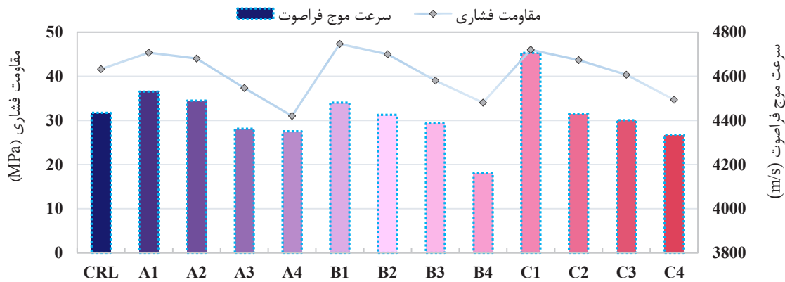
شکل ۱۵. سرعت موج فراصوت و مقاومت فشاری برای همه نمونه‌ها
