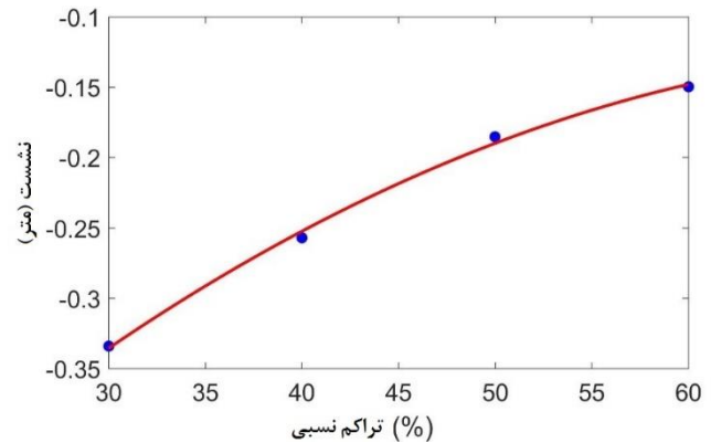
شکل ۱۲. مقایسه نشست زیر پی در تراکم‌های مختلف لایه خاک میانی Fig. 12. Comparison of settlement below the foundation for different densities of the middle soil layer
