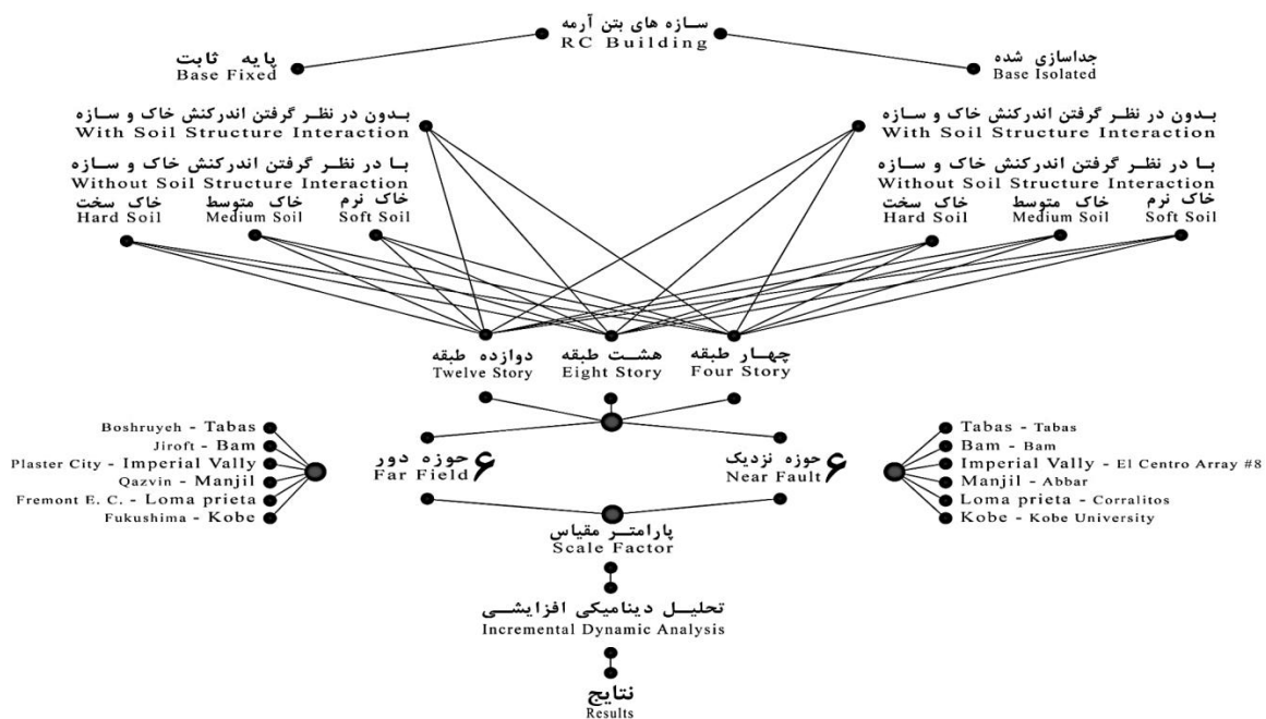
شکل ۴. مسیر انجام تحقیق برای ساختمان های ۴، ۸ و ۱۲ طبقه با و بدون در نظر گرفتن اندرکنش خاک و سازه Fig. 4. Research chart for 4, 8 and 12 story buildings with and without considering the interaction of soil and structures
