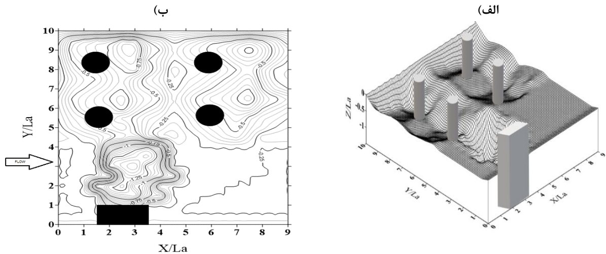
شکل ۱۱. (الف و ب) نمای سه بعدی و خطوط تراز بستر رسوبی با صفحات مستغرق تک ردیفه در آرایش (V-S-2) Fig. 11. View and align lines of experiments with single parallel rows (V-S-2)
