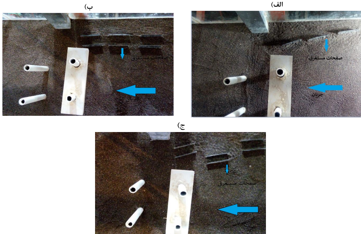
شکل ۸. نمای واقعی: الف) آرایش تک‌ردیفه، ب) آرایش دو ردیفه موازی، ج) آرایش دو ردیفه زیگزاگی Fig. 8. View of reference. a) single parallel rows, b) two parallel rows, and c) two zigzag rows
