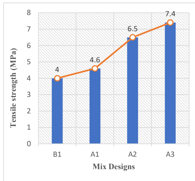
شکل ۴. نمودار مقایسه مقاومت‌های کششی Fig. 4. Comparative diagrams of Tensile strengths
