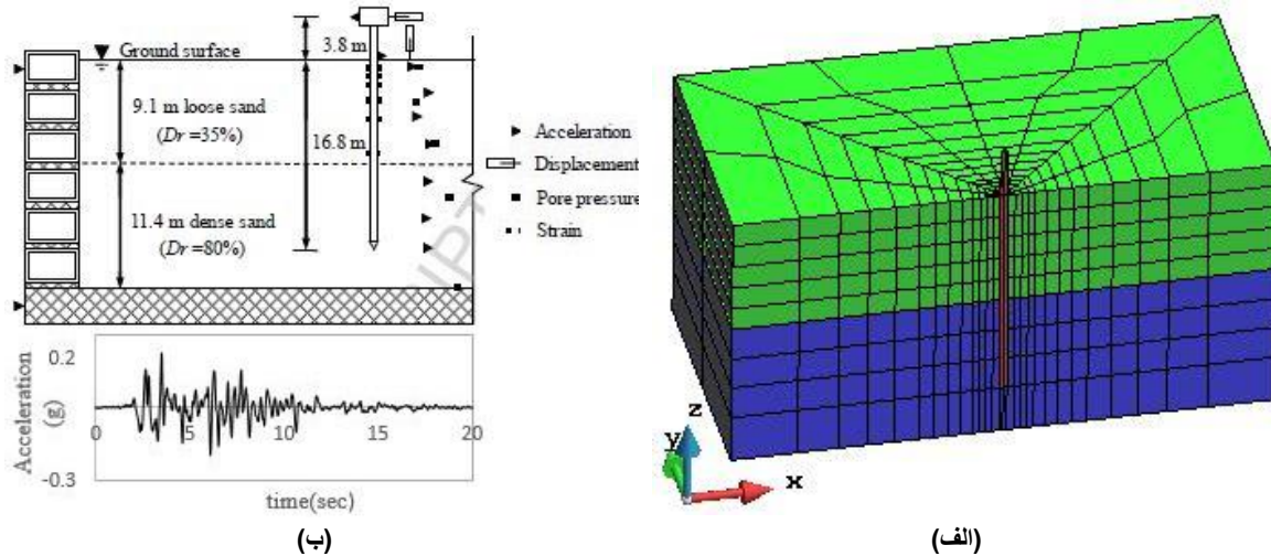
شکل ۶. الف) مدل عددی در نرم افزار اپنسیس، ب) مدل سانتریفیوژ ویلسون نمونه CSP2 [۲۵]
