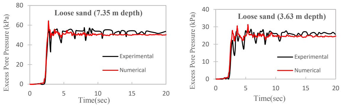
شکل ۷. مقایسه تغییرات فشار آب حفره ای حاصل از نتایج عددی و آزمایشگاهی
