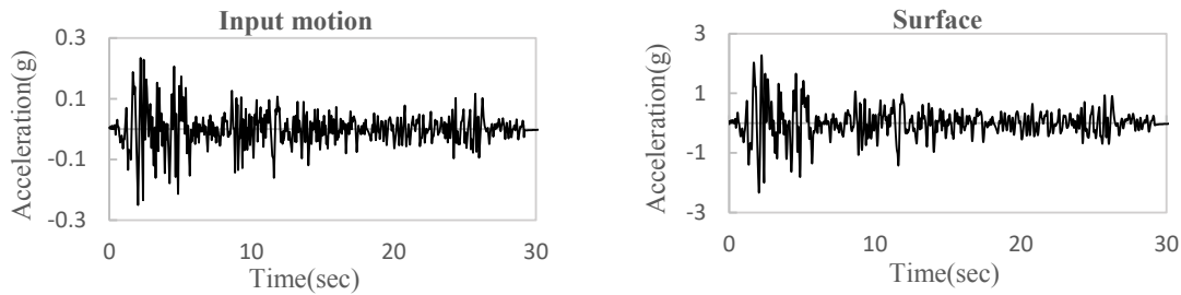
شکل ۱۳. تاریخچه شتاب افقی برای گروه شمع ۱×۱ با A_{rr}=10\% در خاک ماسه ای اشباع یکنواخت در عمق های مختلف تحت رکورد زلزله السنترو Fig. 13. Horizontal acceleration time histories for the 1×1 pile group with A_{rr}=10\% in Uniform saturated Sand Stratum at different depths under the El Centro earthquake
