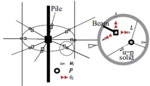
شکل ۳. نحوه اتصال المان شمع به خاک [۱۹]
