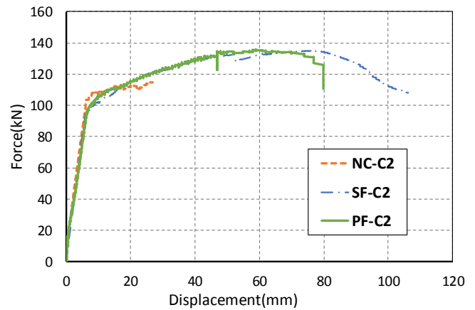
شکل ۲۴. نمودار بار-تغییرمکان تیرهای با خوردگی ۲/۷٪ (گروه C) Fig. 24. Load-displacement curve of corroded beams (7.2%) (Group C)
