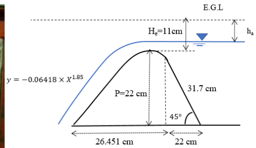
ب: نمایی از سرریز اوجی با شیب وجه بالادست 45 درجه b- A view of ogee weir with inclined upstream face with 45 degrees
