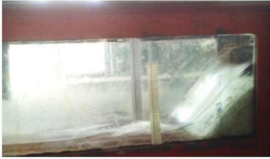
الف: نمایی از سرریز اوجی با وجه بالادست قائم a- View of ogee weir with vertical upstream face
