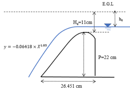
الف: نمایی از سرریز اوجی با وجه بالادست قائم a- View of ogee weir with vertical upstream face
