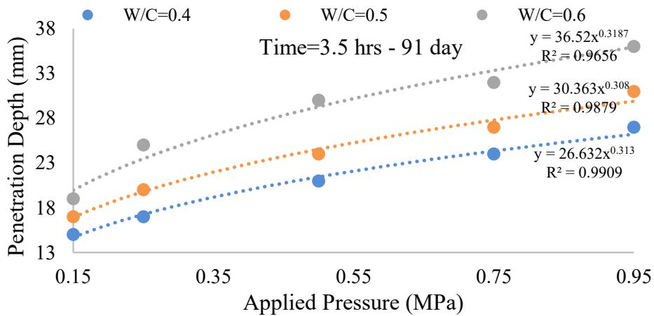
شکل ۱۱. رابطه بین عمق نفوذ و فشار در جهت بتن‌ریزی برای نمونه‌های ۹۱ روزه با نسبت‌های آب به سیمان مختلف (زمان آزمایش ۳/۵ ساعت است). Fig. 11. Relation between penetration depth and pressure in casting direction for the 91-day specimens with different water to cement ratios (test duration is 3.5 hour)
