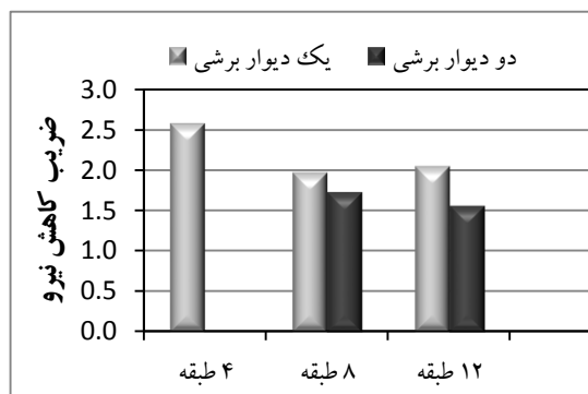
شکل ۸: ضریب کاهش نیرو برای سیستم دوگانه سه دهانه، بارگذاری یکنواخت و اتصال RS
