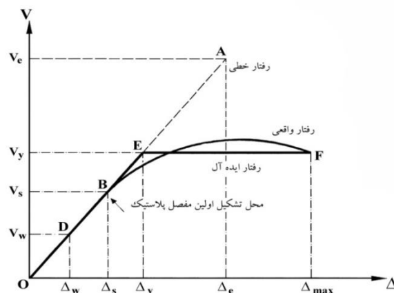
شکل (۱): منحنی پاسخ کلی سازه [۷]
