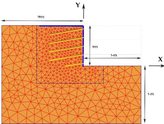
شکل ۸. مدل ۱ در نرم‌افزار اجزای محدود به همراه مش بندی
