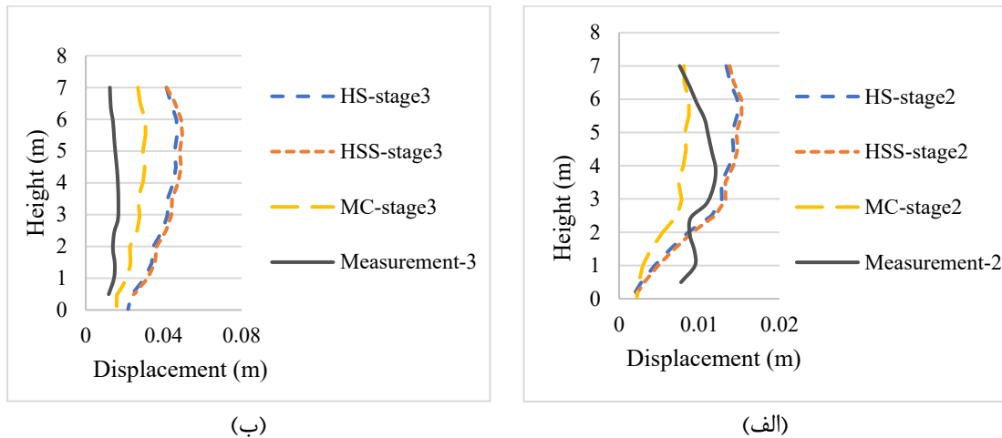
شکل ۱۲. تغییر شکل دیواره گودبرداری (الف) در فاز دوم خاک‌برداری (ب) در فاز سوم خاک‌برداری مدل ۳
