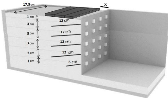
شکل ۵. تصویر شماتیک از جعبه مورد آزمایش در سانتریفیوژ Fig. 5. Schematic of the box test in the centrifuge
