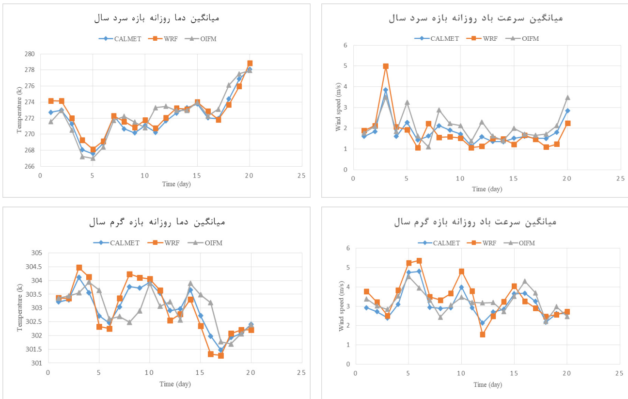
شکل ۴. مقایسه روند تغییرات دما و سرعت باد در دو بازه مدل سازی
