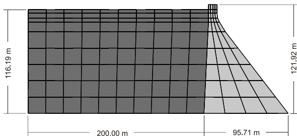
شکل ۱- جزئیات هندسی سیستم سد و مخزن مورد مطالعه
