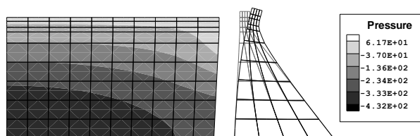
شکل ۵- مود دوم سمت چپ سیستم سد و مخزن وابسته (ضریب بزرگنمایی برای شکل سد معادل ۱۰ ۲ در نظر گرفته شده است.)
