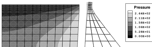
شکل ۲- مود اول راست سیستم سد و مخزن وابسته (ضریب بزرگنمایی برای شکل سد معادل ۱۰ ۵ در نظر گرفته شده است.)
