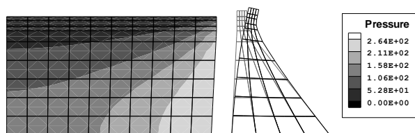
شکل ۳- مود اول سمت چپ سیستم سد و مخزن وابسته (ضریب بزرگنمایی برای شکل سد معادل ۱۰ ۲ در نظر گرفته شده است.)
