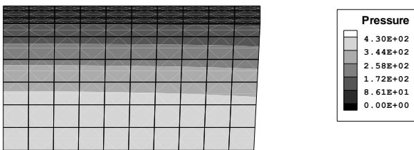
شکل ۱۰- شکل مود اول مخزن
