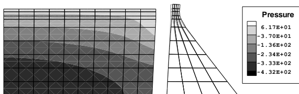
شکل ۴- مود دوم راست سیستم سد و مخزن وابسته (ضریب بزرگنمایی برای شکل سد معادل ۱۰ ۵ در نظر گرفته شده است.)
