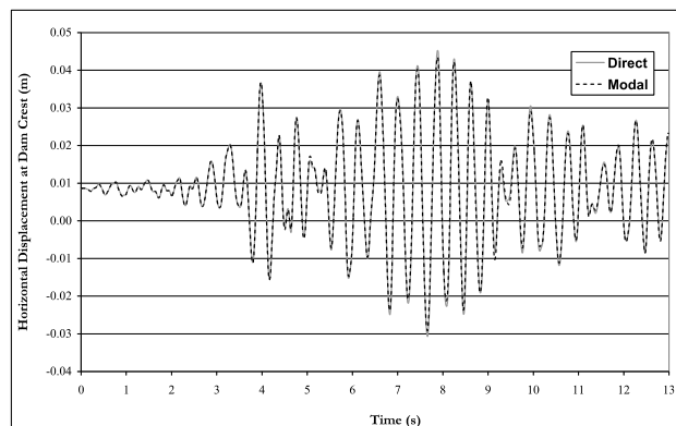
شکل ۱۳- مقایسه پاسخ جابجایی افقی در محل تاج سد به روش مستقیم و مودال غیروابسته- ترکیب D50
