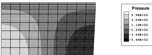
شکل ۱۱- شکل مود دوم مخزن
