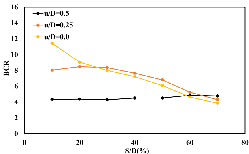
شکل ۱۵. نمودار نسبت ظرفیت باربری برای مقادیر مختلف عمق قرارگیری ژئوسل بطری پلاستیکی برای h/D=1 و b/D=4.5 .
