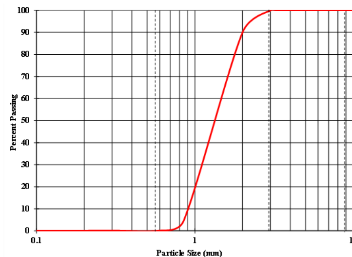
شکل ۳. نمودار دانه بندی و نمای نزدیک از ماسه استفاده شده.
