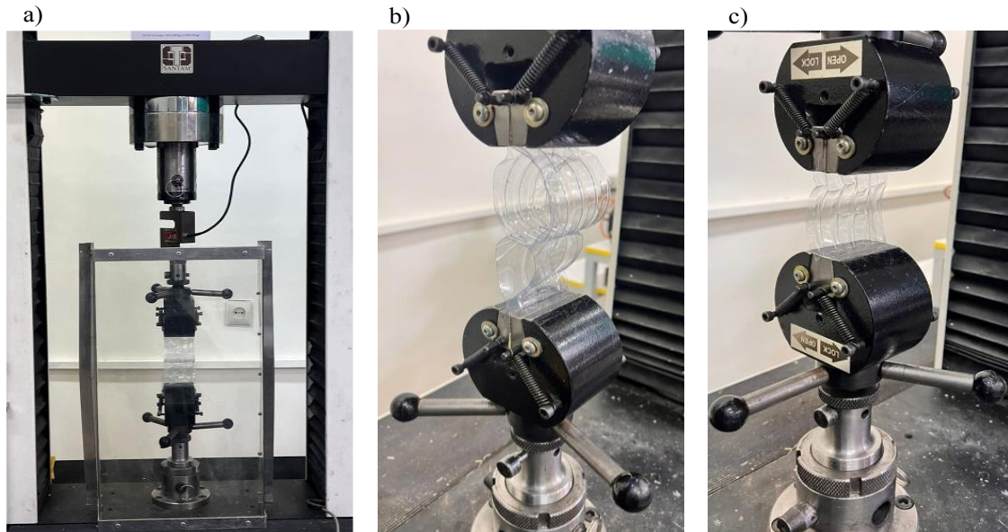
شکل ۵. (a) نمای کلی دستگاه تست یونیورسال، (b) آزمایش کشش اتصال بین بطری ها، و (c) آزمایش کشش بدنه بطری.
