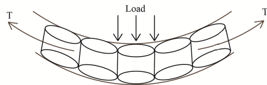
شکل ۱۱. سه مکانیزم مختلف عملکرد ژئوسل [۳۲].
