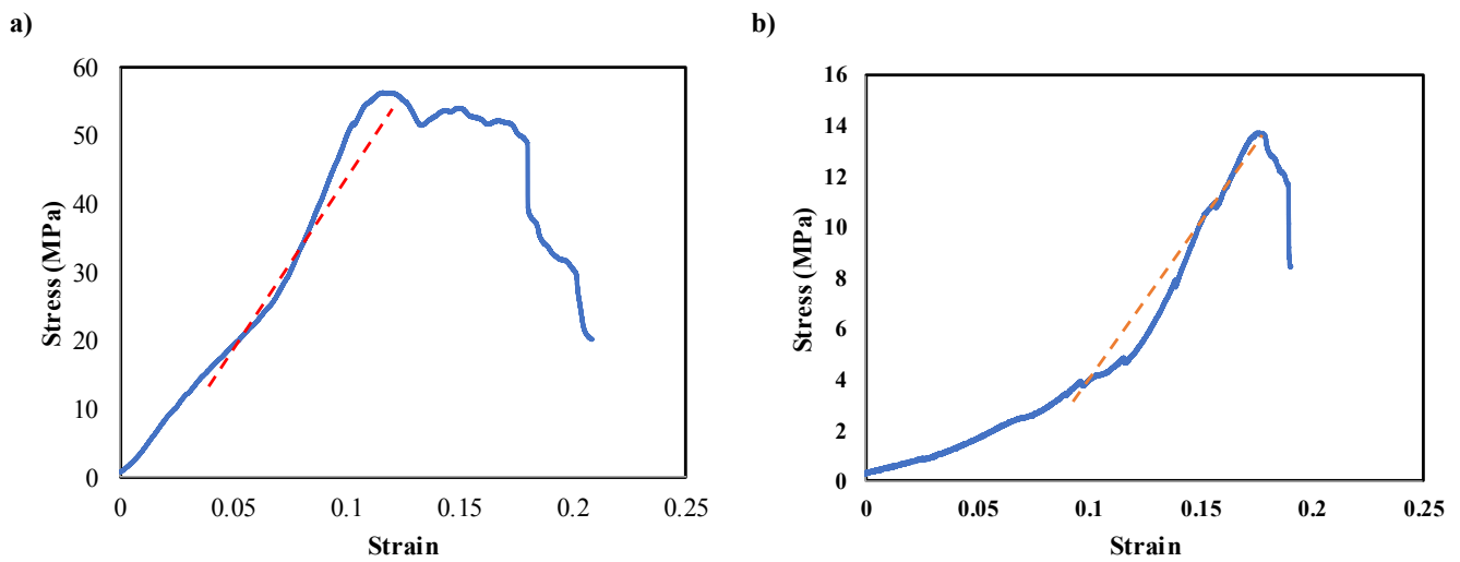
شکل ۶. نمودار تنش- کرنش بطری های پلاستیکی (a) بدنه بطری، (b) اتصال بین بطری ها.
