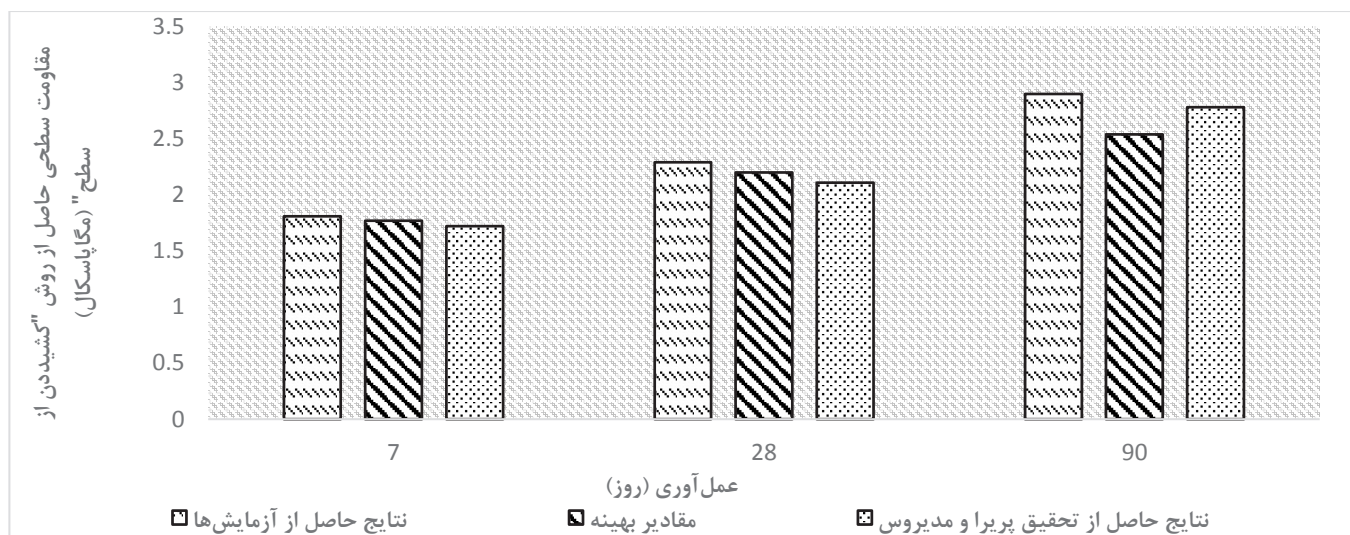
شکل ۱۳. مقایسه نتایج تحقیق حاضر با نتایج تحقیق پیرا و مدیروس
