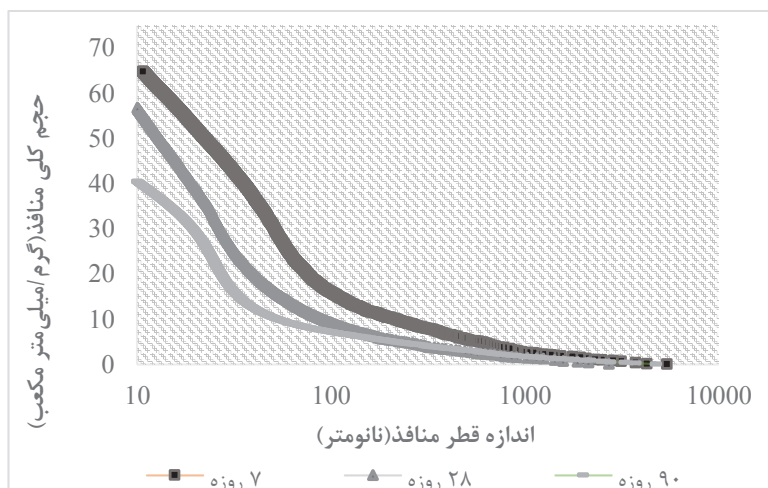
شکل ۷. تغییر در حجم کلی منافذ با افزایش زمان عمل‌آوری
