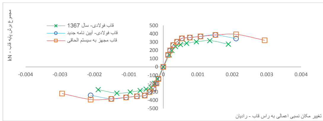
شکل ۲۲. نمودار تغییر مکان نسبی - برش پایه ۸ طبقه
