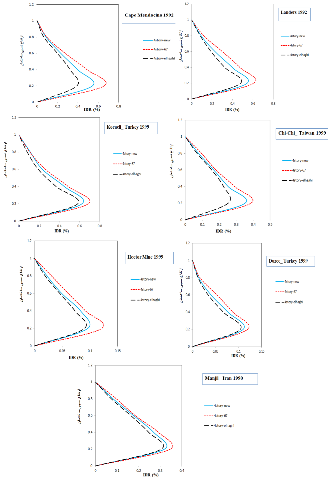
شکل ۳۴. تغییرات IDR - ارتفاع نسبی طبقات سازه‌ی ۴ طبقه تحت شتاب‌نگاشت‌های دور از گسل
