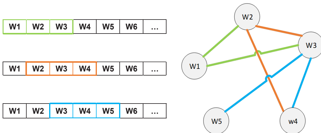
شکل ۲. نحوه گسترش شبکه با پنجره‌ای به طول ۳
