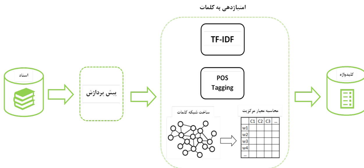
شکل ۱. مراحل استخراج کلمات کلیدی
