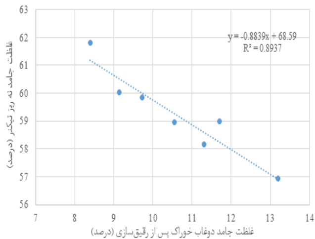
شکل ۶: تاثیر غلظت جامد دوغاب پس از رقیق‌سازی بر غلظت جامد ته‌ریز تیکنرهای باطله مجتمع مس شهربابک
