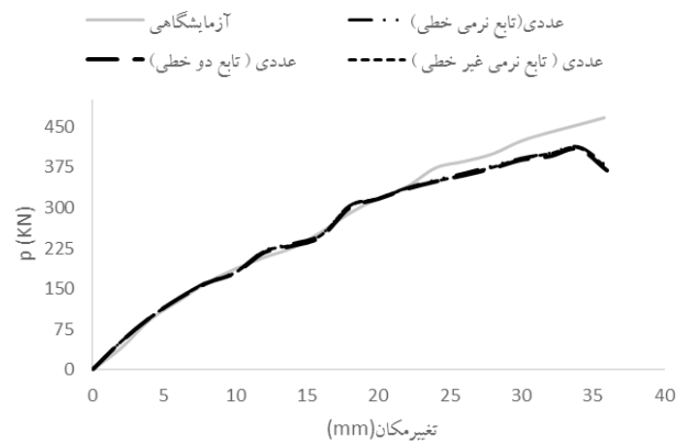
شکل ۱۴: مقایسه نمودارهای بار-تغییر مکان محاسباتی تیر A3 با نمودار آزمایشگاهی
