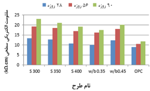
شکل ۸: نتایج آزمایش مقاومت الکتریکی
