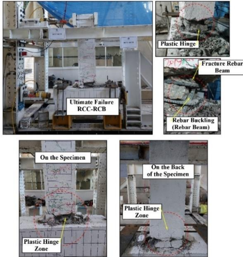
شکل ۱۰. شکست نهایی نمونه RCC-RCB.
