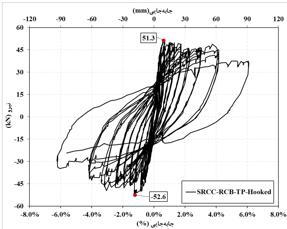
شکل ۱۷. هیستریزیس نمونه SRCC-RCB-TP-Hooked.
