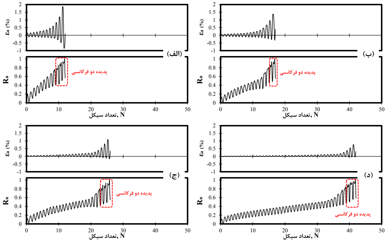
شکل ۸. تغییرات کرنش محوری و فشار آب منفذی نسبی در مقابل تعداد سیکل برای: (الف) زمین سست، (ب) زمین سست بهسازی شده با ستون دانه‌ای، (ج) ستون دانه‌ای با روکش ژئوگرید نوع ۱، (د) ستون دانه‌ای با روکش ژئوگرید نوع ۲
