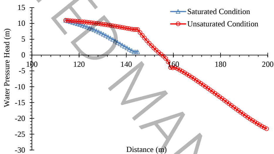
شکل ۱۶. توزیع بار فشار در مقطع افقی یک (Section 1) برای جریان اشباع و غیر اشباع
