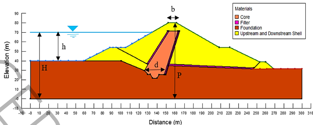
شکل ۴. طرح کلی از سد شبیه‌سازی شده در نرم‌افزار Fig. 4. Dam Model Simulated in the Software
