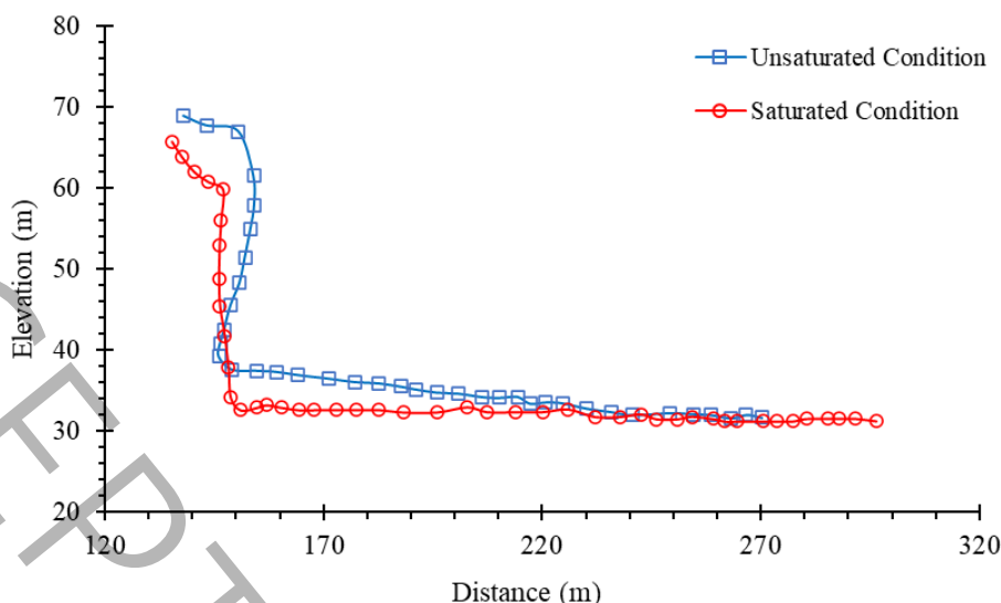
شکل ۱۰. موقعیت خط فریاتیك در بدنه سد خاكي برای جریان اشباع و غیر اشباع
