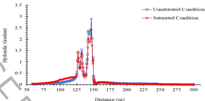
شکل ۱۳. تغییرات گرادیان هیدرولیکی در بدنه سد خاکی
