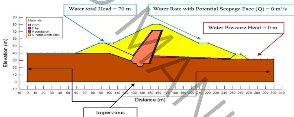
شکل ۵. شرایط مرزی تعریف شده برای هندسه سد خاکی گیلان‌غرب Fig. 5. Defined Boundary Conditions for the Geometry of Gilan Gharb Earth Dam
