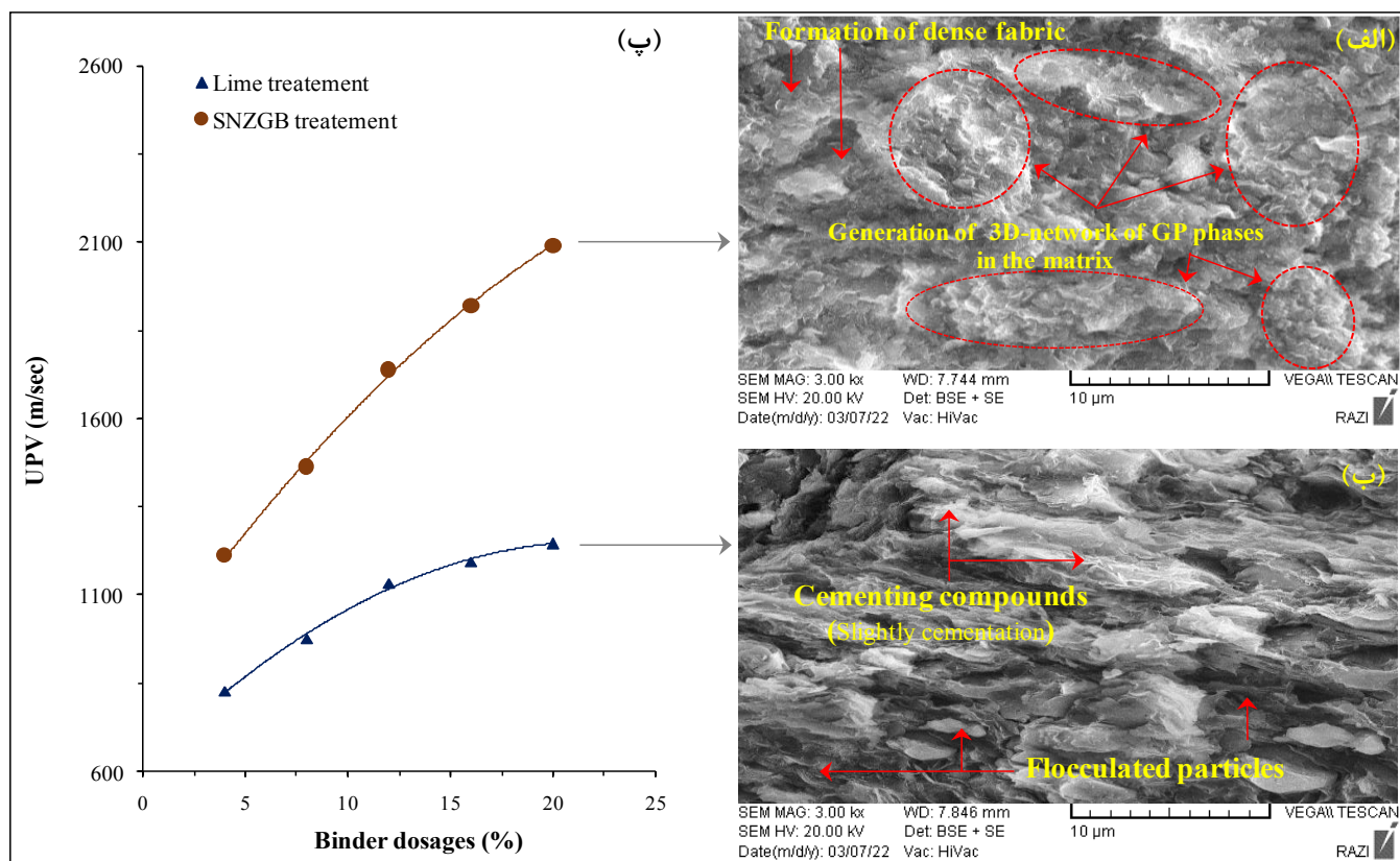
شکل ۷. مقایسه (الف و ب) ریزساختار و (ت) تغییرات سرعت پالس الیتراسونیک مصالح در حضور SNZBG نسبت به آهک
