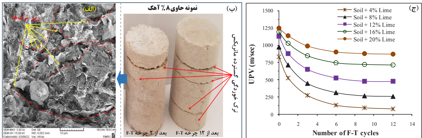
شکل ۴. (الف) تشکیل ریز-ترک‌ها، (ب) ناپایداری ظاهر، و (ج) تغییرات سرعت پالس التراسونیک بر اثر مجاورت خاک با چرخه یخ-ذوب
