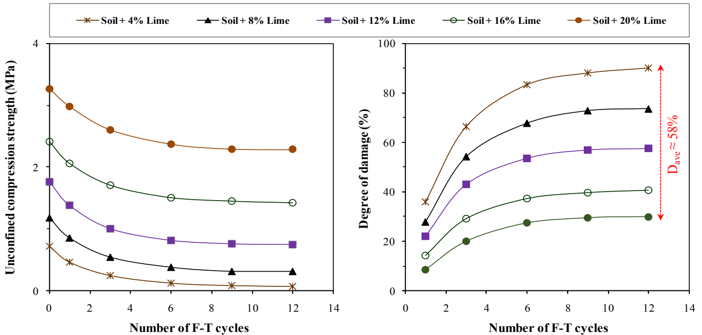
شکل ۲. تاثیر چرخه یخ و ذوب بر خصوصیات مکانیکی خاک حاوی آهک بعد از ۲۸ روز عمل‌آوری
