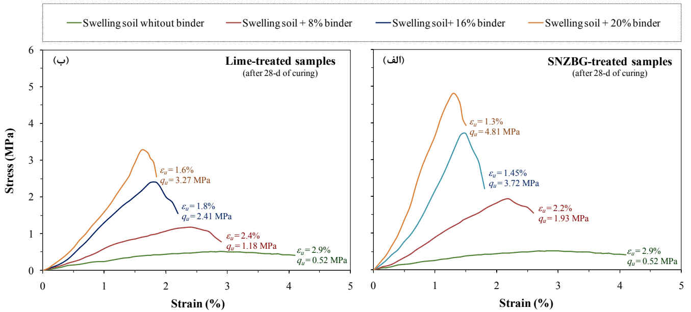
شکل ۸. پاسخ تنش-کرنش مصالح بعد از ۲۸ روز نگهداری در حضور مقادیر مختلف (الف) SNZBG و (ب) آهک
