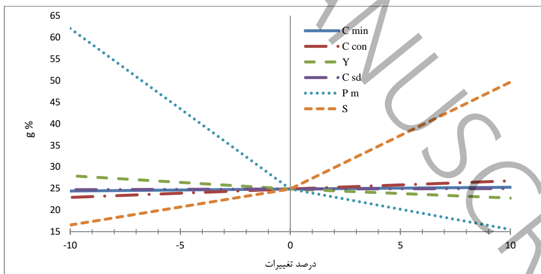
شکل ۳. تحلیل حساسیت عیار حد نسبت به هزینه‌ها
