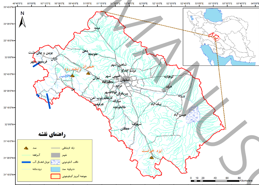
شکل (۲) - موقعیت حوضه آبریز گاوخونی
