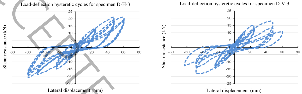
شکل ۱۳: چرخه‌های هیسترسیز بار-تغییرمکان نمونه‌ها
