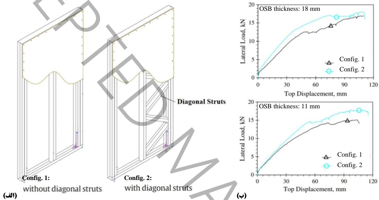
شکل ۱: الف- جزئیات پانلهای با و بدون مهاربند قطری، ب- تأثیر وجود مهاربند قطری روی منحنی پاسخ بار-تغییرمکان [۸]
