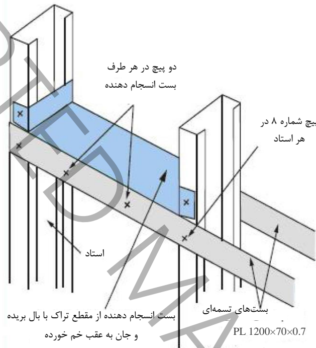
شکل ۱۰: اتصال بست‌های تسمه‌ای، انسجام دهنده و استاداها [۶]
