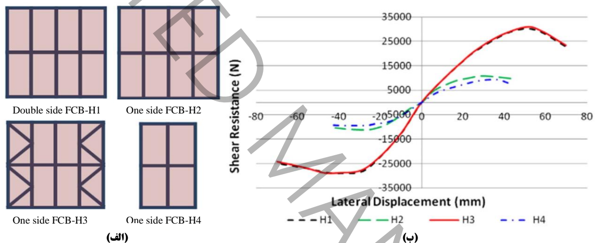
شکل ۲: الف- پیکربندی نمونه‌ها، ب- منحنی پوش هیسترسیز [۱۳]
