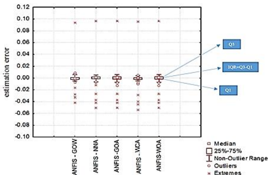
شکل ۷. نمودار جعبه‌ای توزیع خطای تخمین دبی ورودی سد در مرحله آزمون برای همه مدل‌ها، ۲۵٪ چارک پایین خطاها، ۷۵٪ چارک بالای خطاها.
