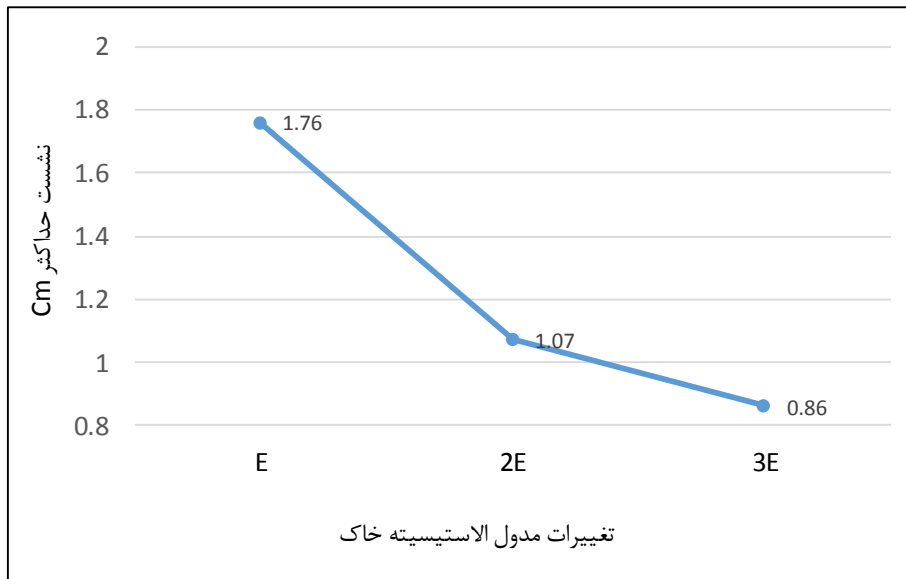
شکل ۱۹. تغییرات جابه‌جایی‌ها با تغییر مدول الاستیسیته خاک
