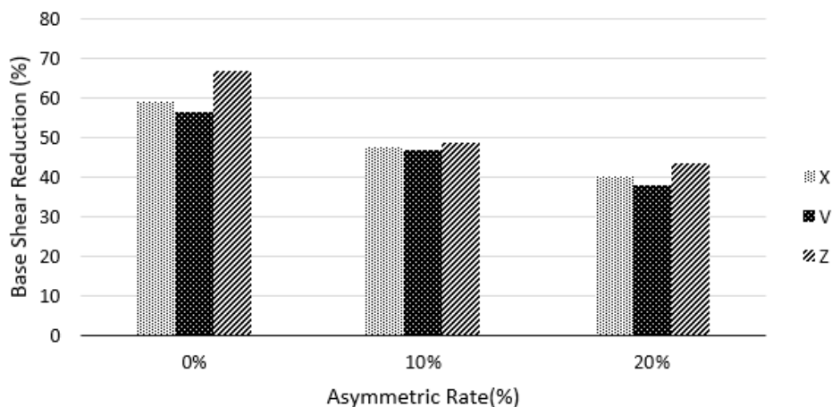
شکل ۱۶. مقدار متوسط کاهش برش پایه در سازه ۱۰ طبقه با مهاربندهای X, V, Z، پایه (FB), (IB) و نامتقارنی (A0%, A10%, A20%)
