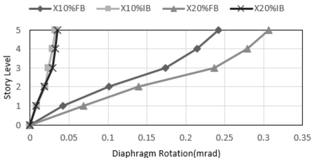
شکل ۱۳. مقدار میانگین دوران طبقات سازه با مهاربند V با پایه (IB) و (FB) با نامتقارنی (A10%, A20%) Fig. 13. Average sotry rotation of 5-story structure (base-isolated and fixed base) with V brace & different asymmetric values (A10%, A20%)
