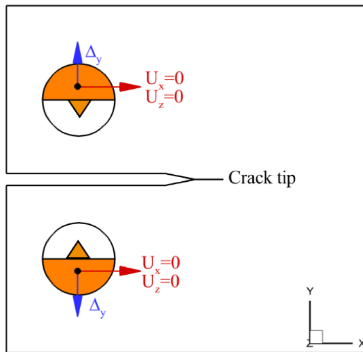
شکل ۴. الف) مش بندی مدل عددی و محل المان تماسی، ب) شرایط مرزی
