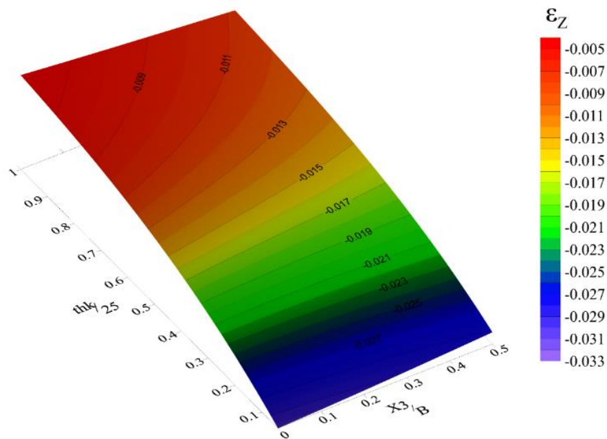
شکل ۶. کرنش در راستای عمود بر صفحه برای ضخامت های مختلف و در طول ضخامت در انتهای بارگذاری Fig. 6. Strain perpendicular to the plane for different thicknesses and along thickness length
