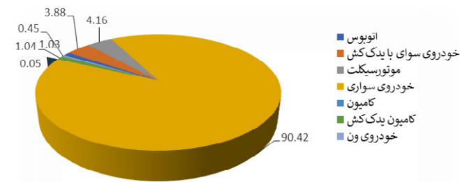
شکل ۳. ترکیب ناوگان عبوری در پل صدر تهران
