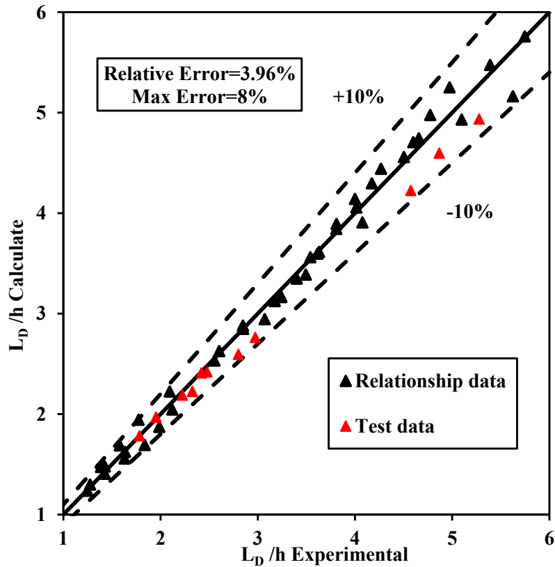
شکل ۸. مقایسه مقادیر آزمایشگاهی \frac{L_D}{h} با مقادیر محاسباتی
