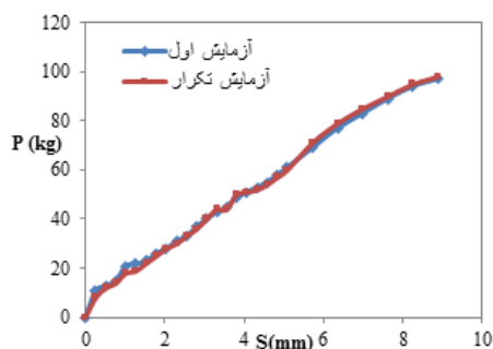
شکل ۷: تکرار پذیری نمونه‌های غیر مسلح
