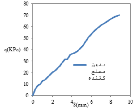
شکل ۹: نمودار تنش-نفوذ سنبه برای نمونه غیر مسلح
