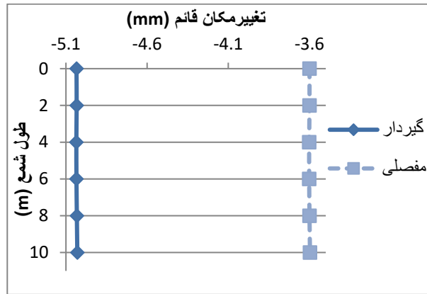
شکل ۸. بررسی اثر نحوه اتصال شمع و سرشمع بر توزیع تغییرمکان قائم در طول شمع
