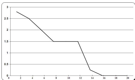
شکل ۳: روند بدست آمدن ضریب اطمینان آستانه لغزش (FS=1) Fig. 3. Trend to obtain slip threshold confidence coefficient (FS = 1)
