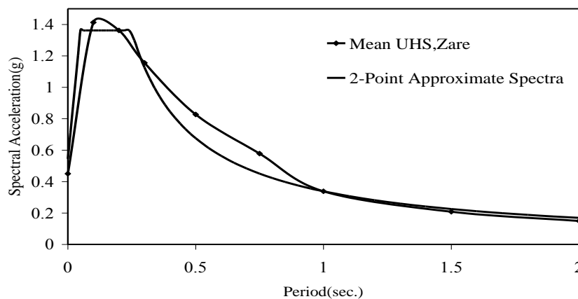
شکل (۷): طیف طرح دو پارامتری و طیف خطر یکنواخت افقی میانگین، با شرایط ساختمانی سنگ احتمال وقوع ۵۰ / ۱۰٪، میرایی ۵٪، روابط کاهندگی زارع (۱۹۹۹، ۲۰۰۶)
