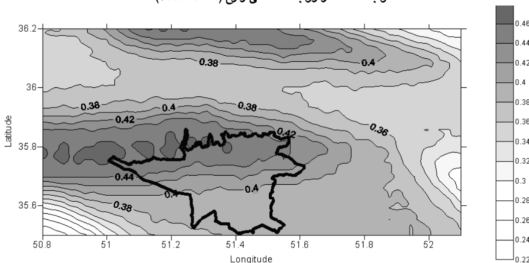
شکل (۴): نقشه شتاب افقی حداکثر زمین (PGA) یا شتاب طیفی در زمان تناوب صفر ثانیه (g)، با احتمال وقوع ۱۰٪ در طول ۵۰ سال و با استفاده از روابط کاهندگی (Campbell & Bozorgnia (2003, 2006)
