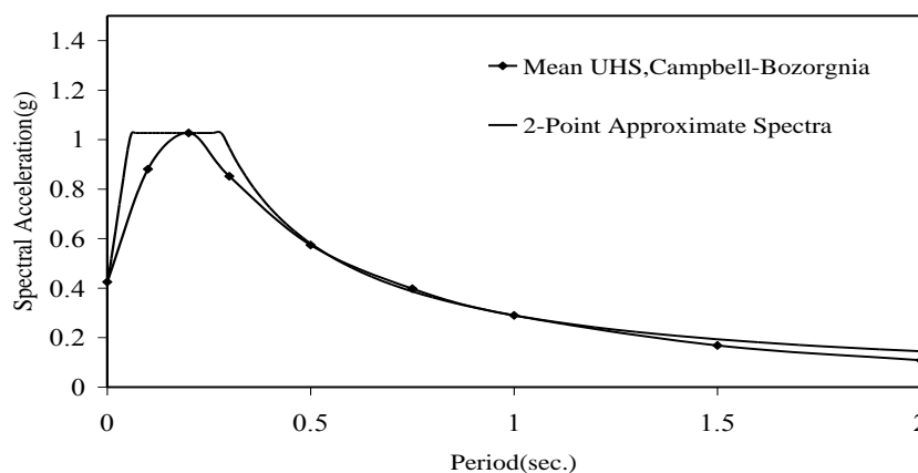
شکل (۸): طیف طرح دو پارامتری و طیف خطر یکنواخت افقی میانگین، با شرایط ساختمانی سنگ احتمال وقوع ۵۰ / ۱۰٪، میرایی ۵٪، روابط کاهندگی Campbell & Bozorgnia (2003, 2006)
