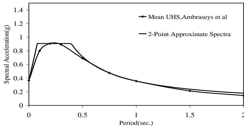
شکل (۶): طیف طرح دو پارامتری و طیف خطر یکنواخت افقی میانگین، با شرایط ساختمانی سنگ احتمال وقوع ۵۰ / ۱۰٪، میرایی ۵٪، روابط کاهندگی Ambraseys et al. (1996, 2003)
