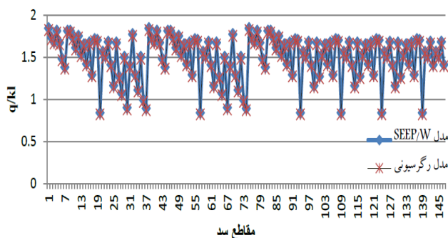
شکل (۴): نمودار تغییرات q/kl در مقاطع مختلف
